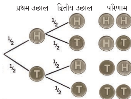
चित्र 7.6 — एक निष्पक्ष सिक्का दो बार उछालने पर संभावित परिणाम दर्शाता वृक्ष आरेख
